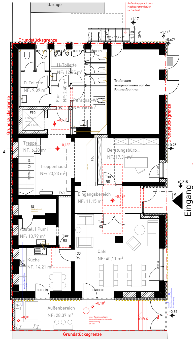
Jugendzentrum Herxheim | Erdgeschoss + Südansicht
